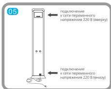
05 Выберите место для подключения к сети переменного напряжения 220 В (вверху или внизу). Намотайте катушку питания. Произведите настройки. Закрепите изделие к полу с помощью крепежных винтов. Изделие готово к работе.
